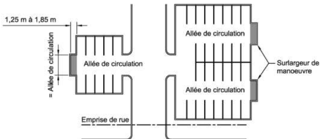
Figure XXI.1 Surlargeur de manœuvre
